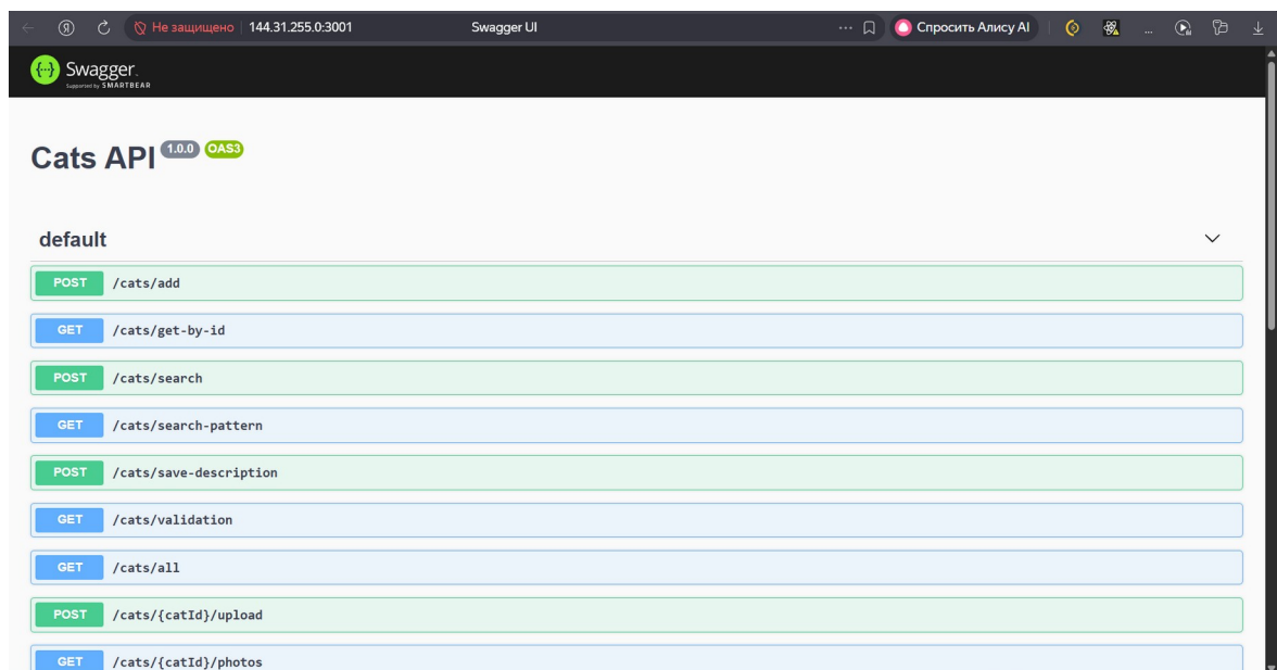
Рисунок 2 – открытый Swagger
